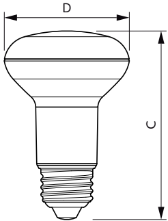
R20 120V 5-45W 450lm 90D 3000K E26 D
