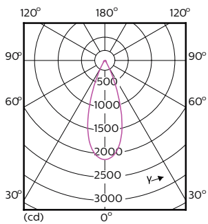
PAR30L 120V 12-75W 900lm 40D 3000K E26 D
