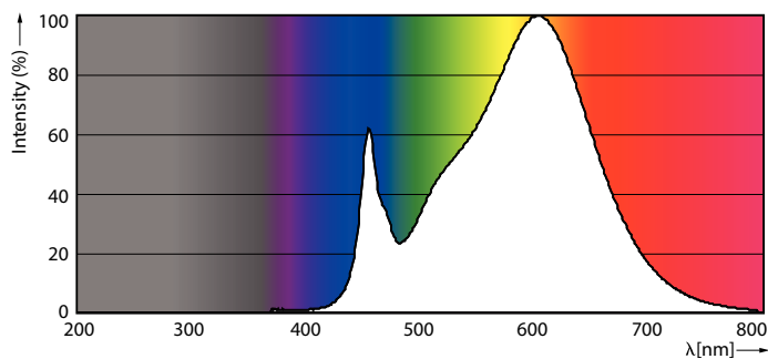
LEDtube_G13_830-POC
