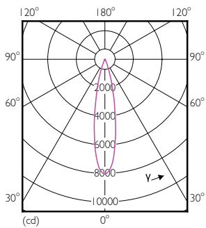
PAR38 17W 1300lm 25D 4000K E26
