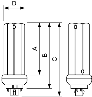
PL-T 42W/835/A/4P/ALTO
